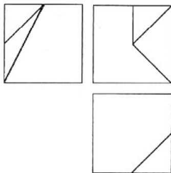
7 Dibuja en caballera o axonometría
