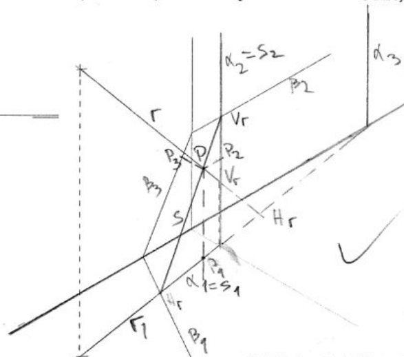
11 Halla el punto de intersección de R con el plano A
